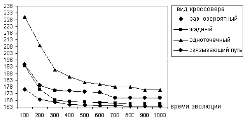
в) равновероятная селекция, p_m = 0,02
