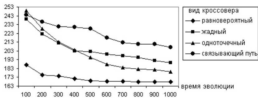
б) селекция "лучший и случайный", p_m = 0,02
