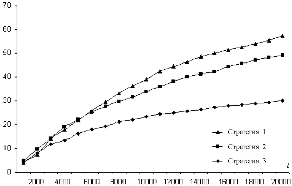
Рис. 13. Частота получения точного решения для l = 50
