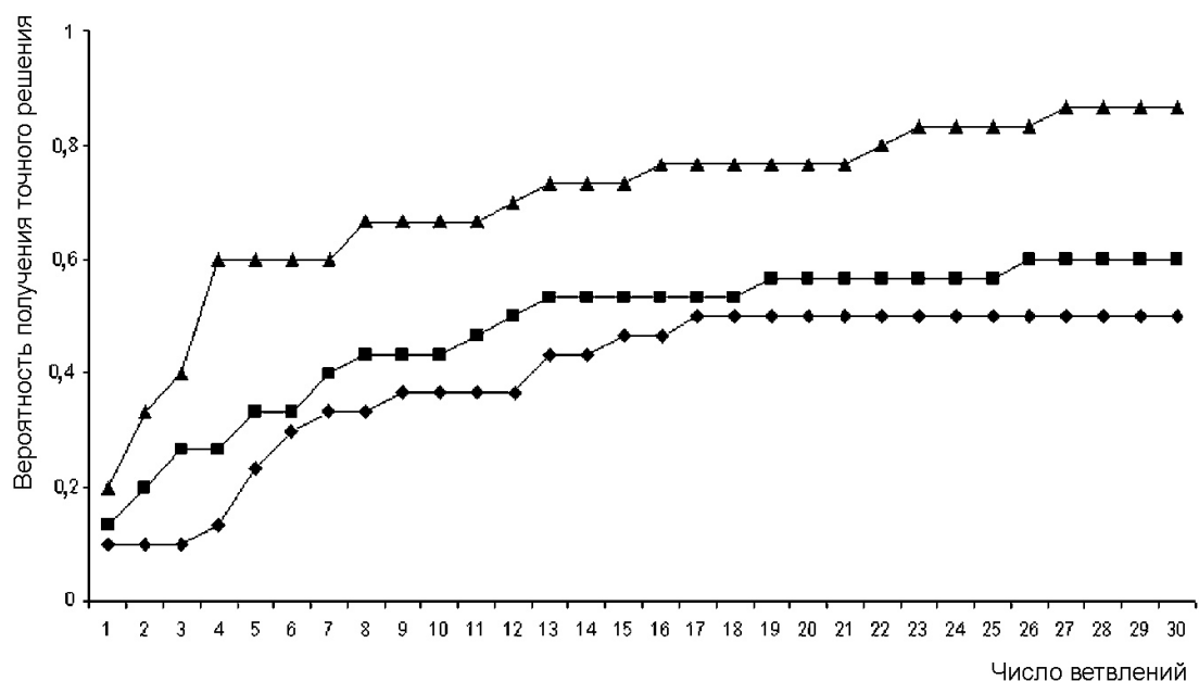
б) изменение частоты получения точного решения Pr(\varepsilon = 0)
