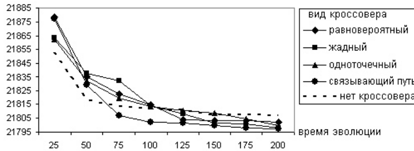
е) турнирная селекция, p_m = 0,5 , класс Euclidean
