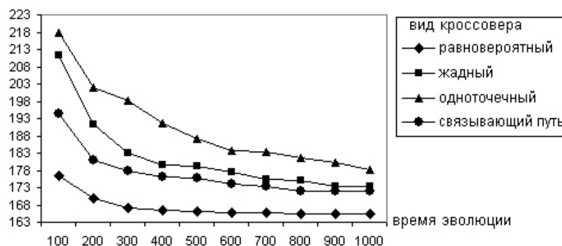
а) турнирная селекция, p_m = 0,02
