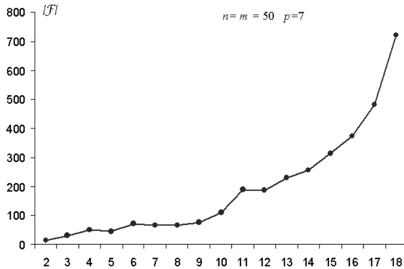
Рис. 25 Зависимость размера семейства \mathcal{F} от параметра r при фиксированном p ( p = 7 ).
