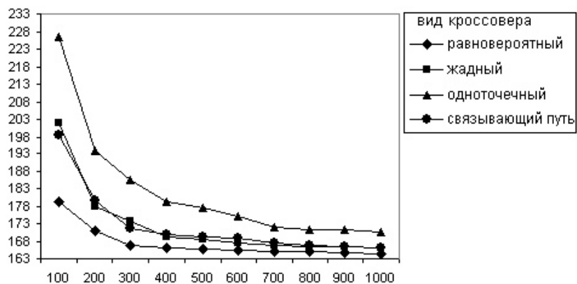
г) турнирная селекция, p_m = 0,1
