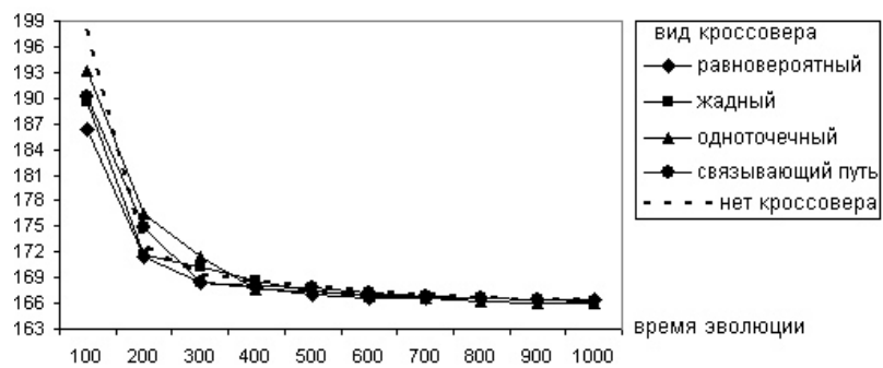
д) турнирная селекция, p_m = 0,5
