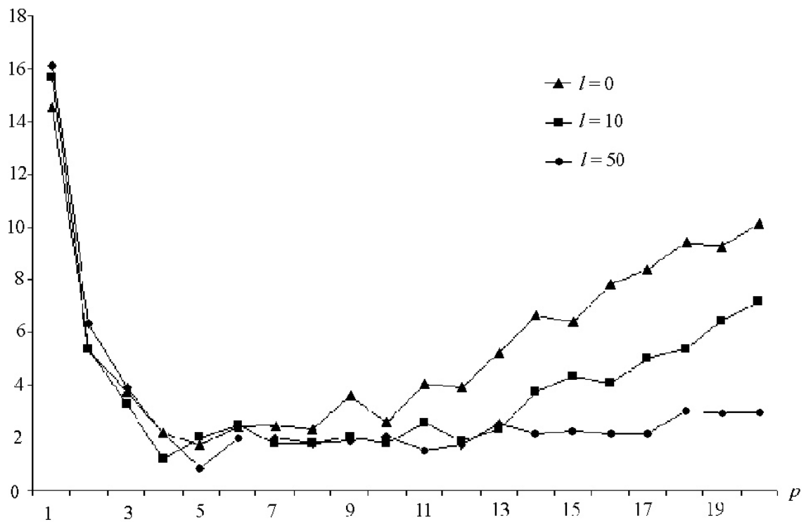
Рис. 12. Изменение \varepsilon(p) при T = 20000
