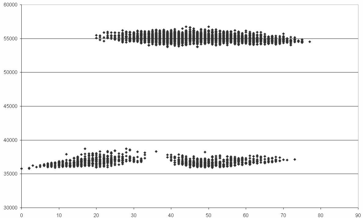
Рис. 22. Взаимное расположение кластеров
