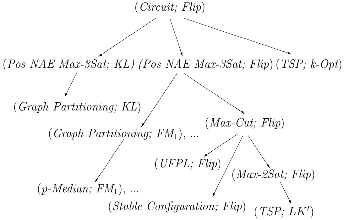
Рис. 16. PLS-полные задачи
