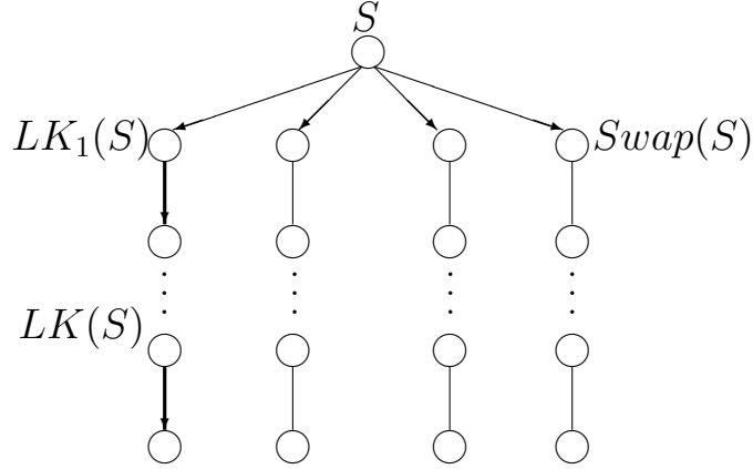
Рис 17. Окрестность TreeLK(S)
