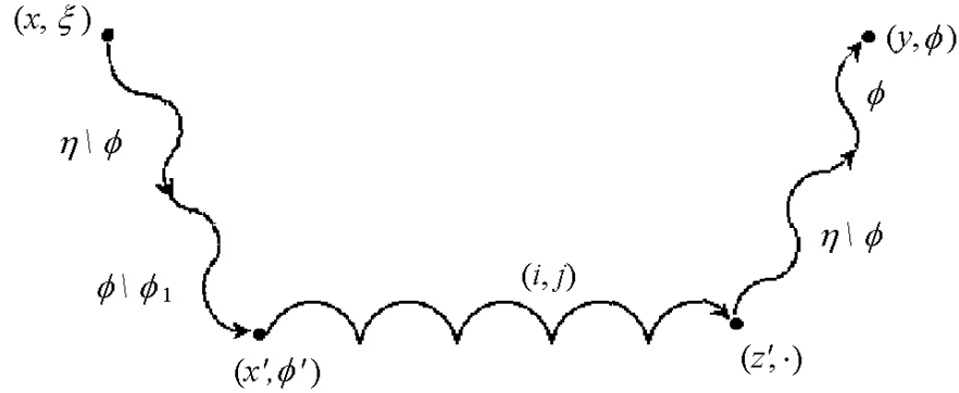
Рис. 11. Путь от (x, \xi) до (y, \phi)
