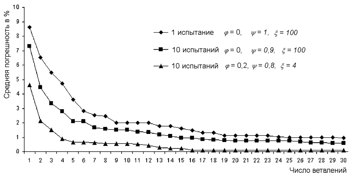
а) изменение средней относительной погрешности M(\varepsilon)
