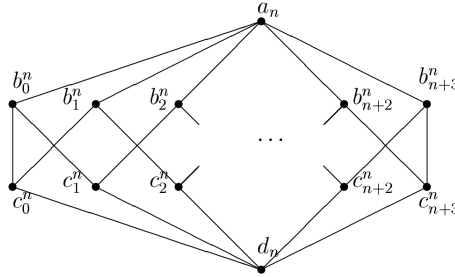
Рис. 1. Решетка R_n .
