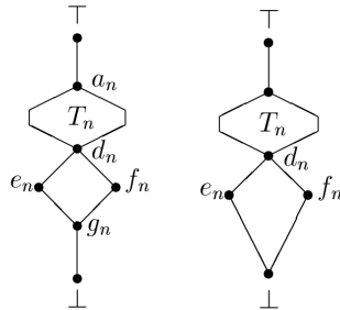
Рис. 2. Фрагменты L .
