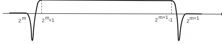
Рис. 2. Срезающая функция.
